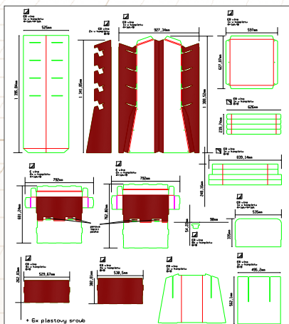
Příklad technického výkresu stojanu
